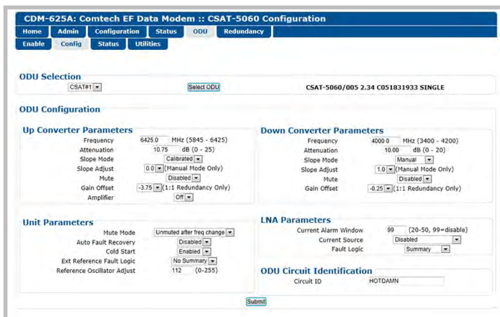
Figure 10-9. ODU | Config page (CSAT-5060)
